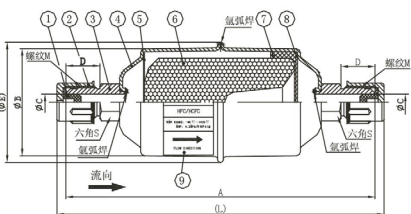
螺口 Thread
