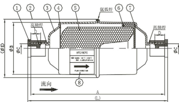
焊口 Soldering
